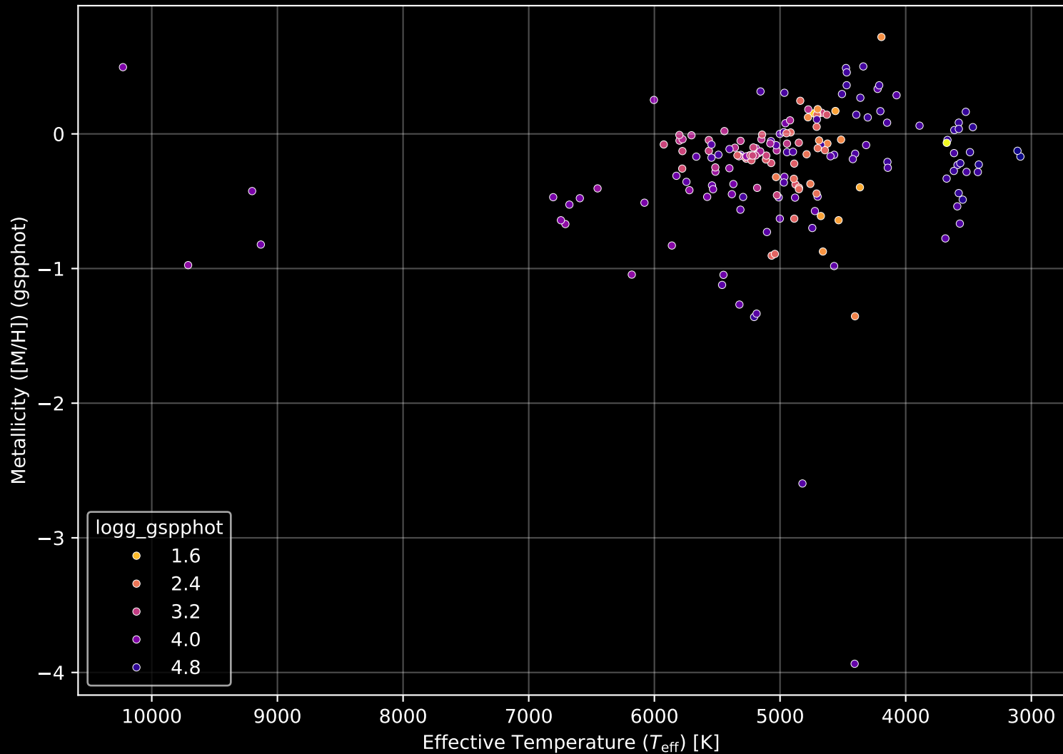
APOGEE DR17 Field: [170-23-O] Stellar Population Parameters (n= 181)
